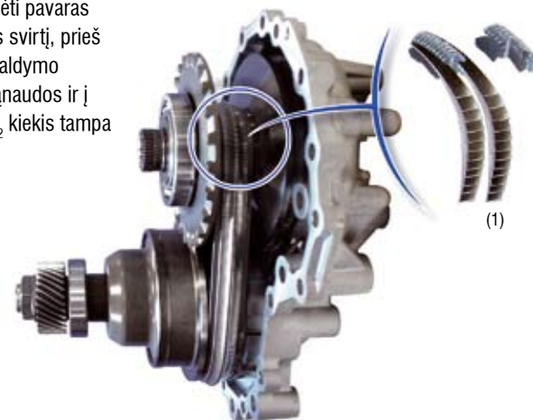
(1) Du kintamo diametro skriemuliai, esantys mechanizmo viduje, yra sujungti metaliniu dirželiu.
